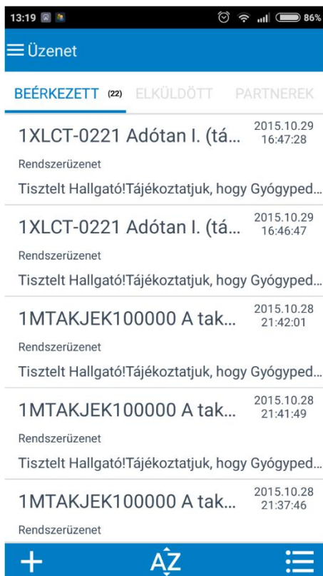
Android
