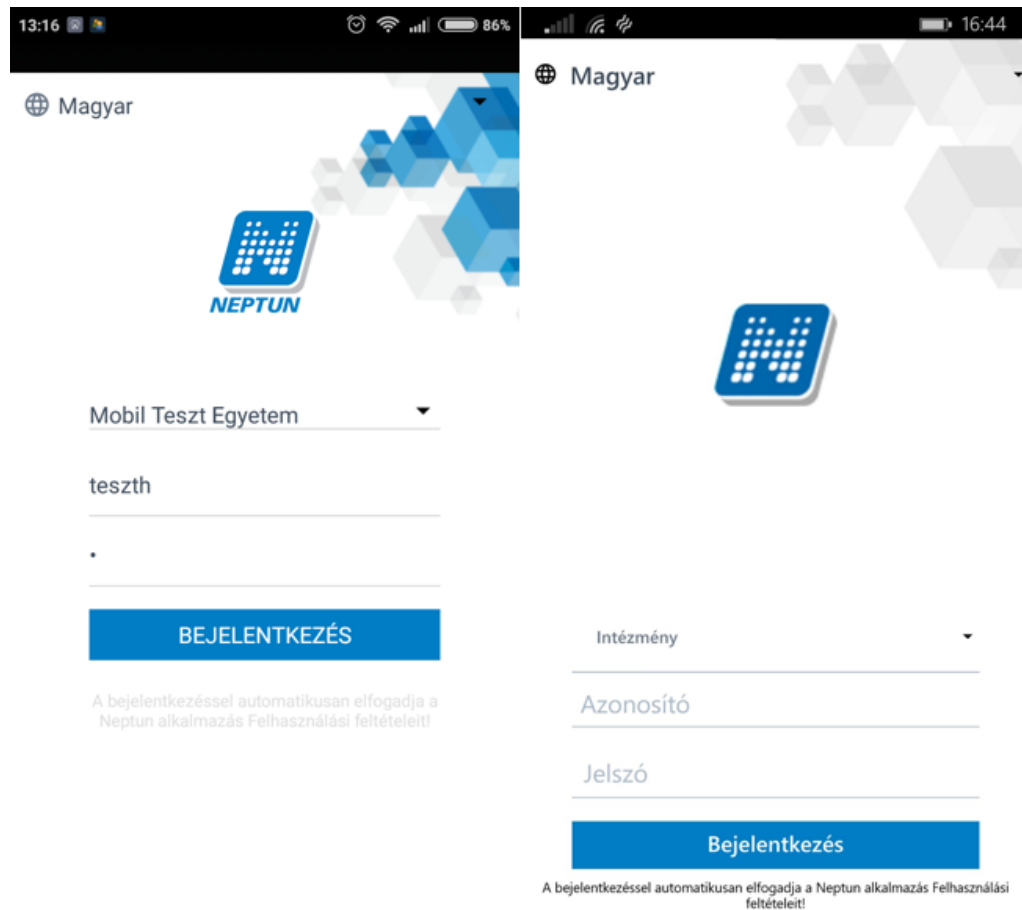
Android
